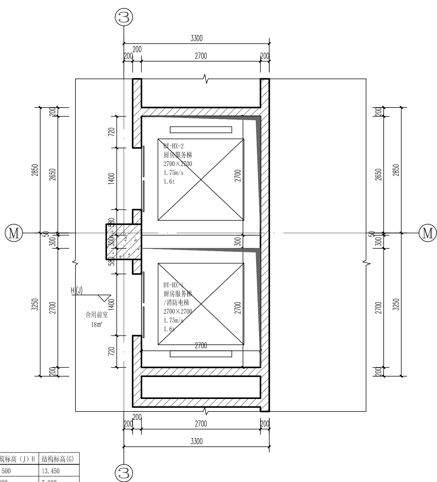
DT-HX-1~2 地下二层~三层平面
