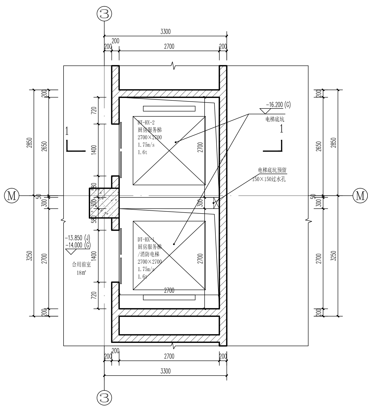
DT-HX-1~2 地下三层平面
